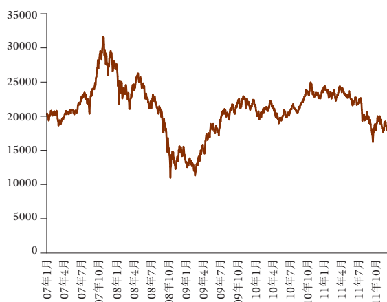
恒指 (01/2007 – 12/2011)
