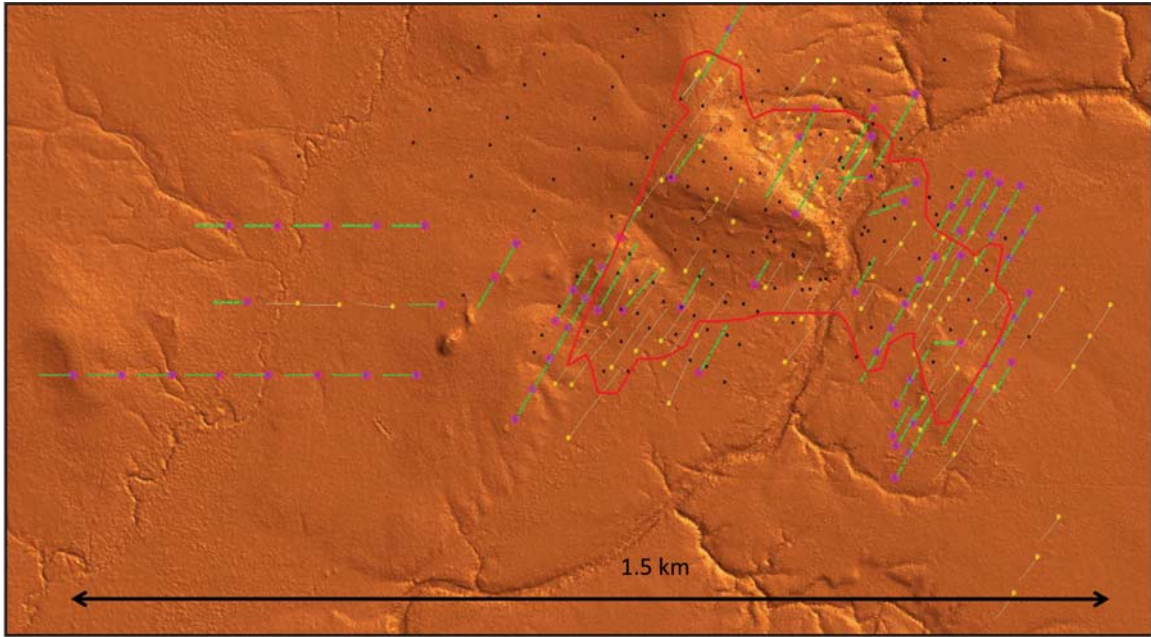
圖3：計劃中二零一一年第一期鑽探計劃及覆蓋於數碼地勢模型的礦務資源估計周界（紅色）。鑽探已於二零一一年五月展開。載於本公告現有礦務資源估計以西已目視觀察到的礦務資源令人鼓舞。
