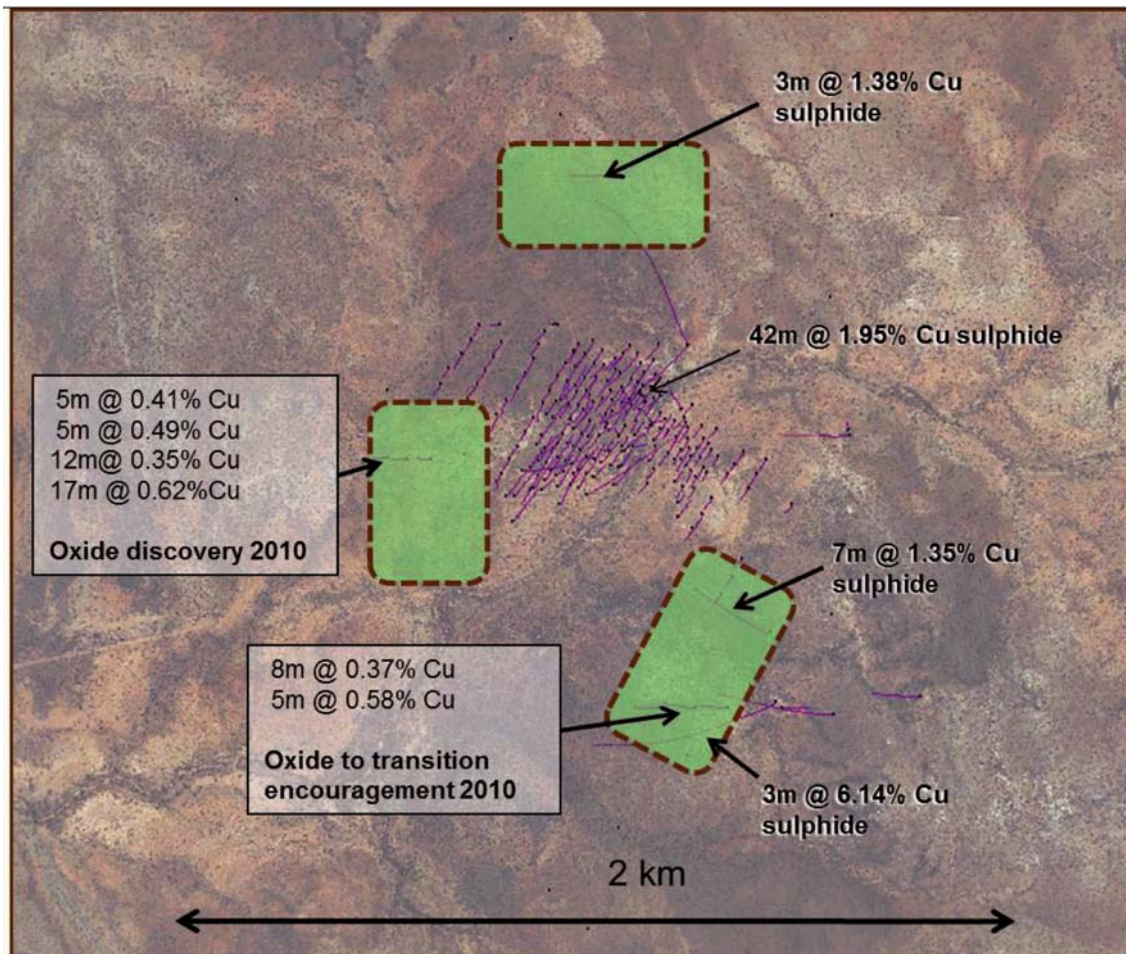
圖4：部份以往重大穿切，顯示中科礦業Lady Annie營運勘探於二零一一年測試的進一步潛在儲量。
