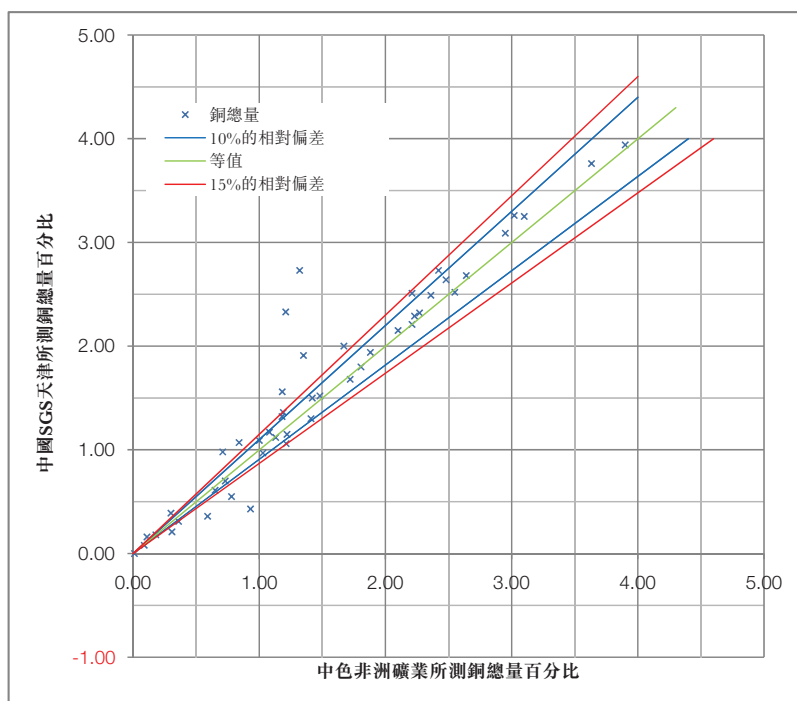
圖6-20：Chambishi 東南礦岩芯礦漿複樣檢測結果
