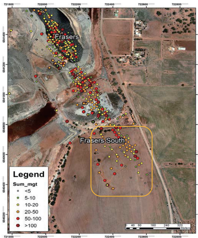
圖2－Frasers 金礦分佈圖，黃框是此次鑽探的範圍。
