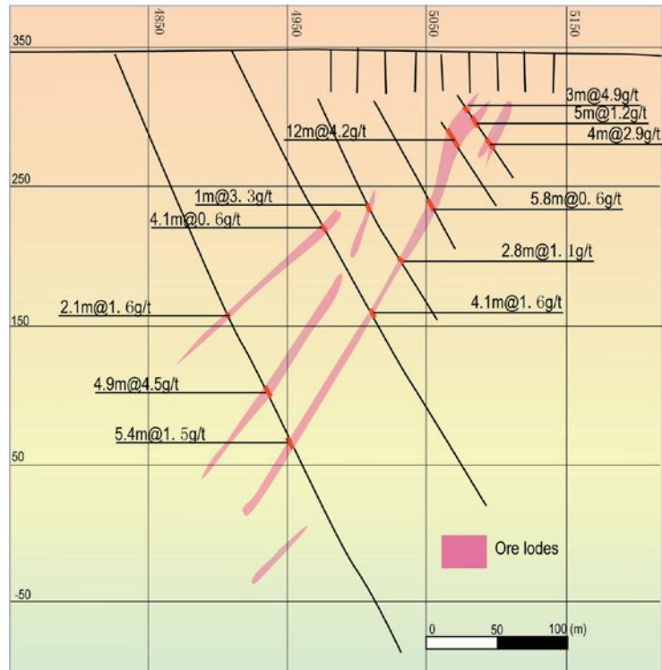
圖3—Frasers 金礦南段11140N 線鑽探剖面圖
