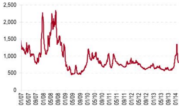
图 4：2010~2014 年 BDTI 走势
