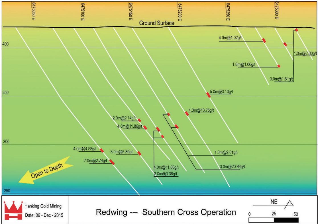
圖2－罕王黃金REDWING金礦剖面圖
