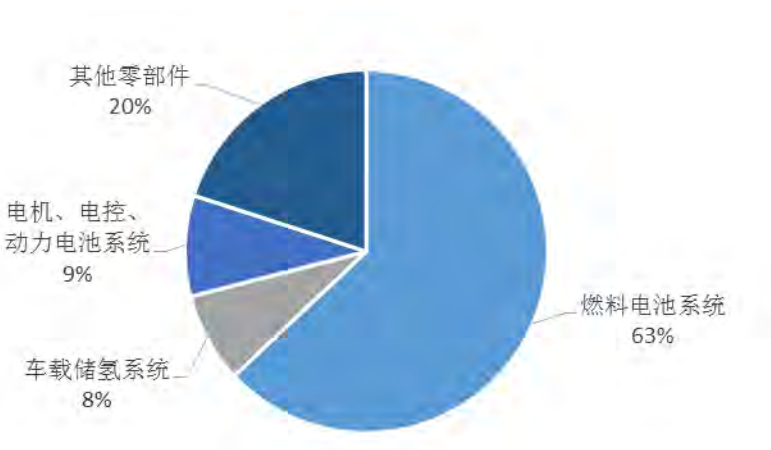
图：燃料电池汽车成本构成
