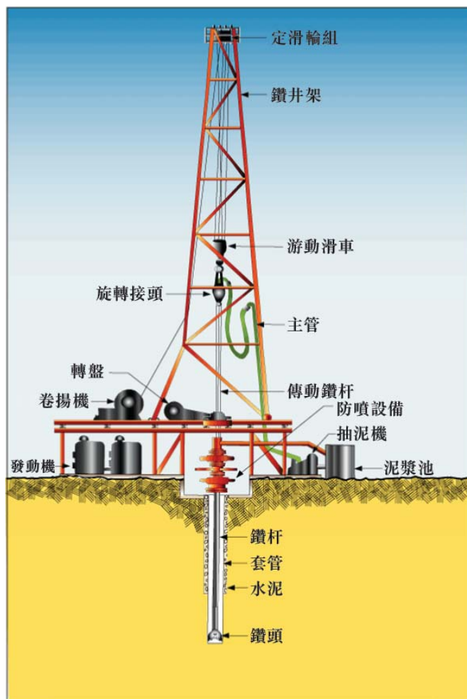
圖一：陸上鑽油台圖解
