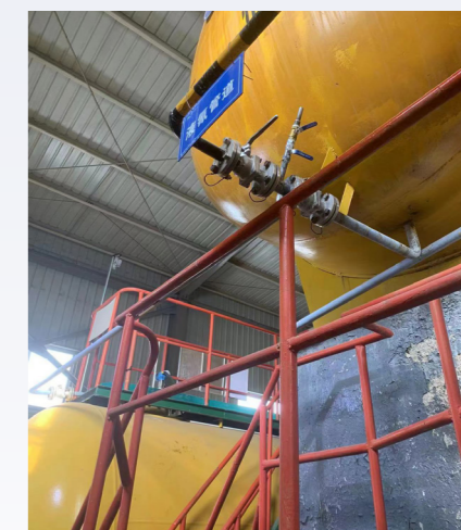
整改後的液氫庫液氫管道閘門
