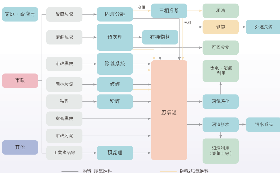
有機垃圾綜合處理流程示意圖
